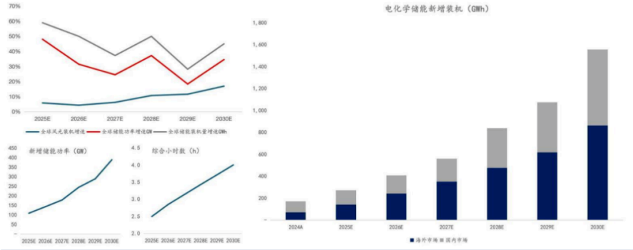
图表30：全球储能新增装机量需求预测汇总
